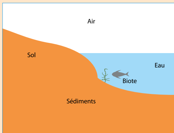
Compartiments environnementaux
